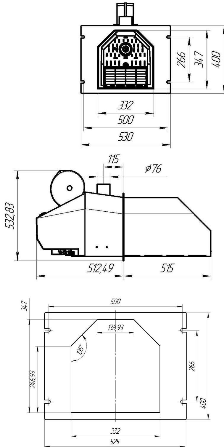
Рис. 1. Габаритні та приєднувальні розміри пальника. 250 кВт.
